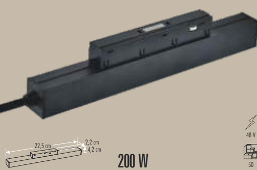
CT-5971 RENO MAGNETIC TRAFO
